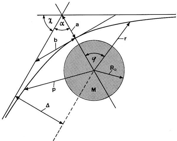
Fig. 1: Hyperbelbahn im KEPLER-Problem. Zentralkörper mit der Masse M
